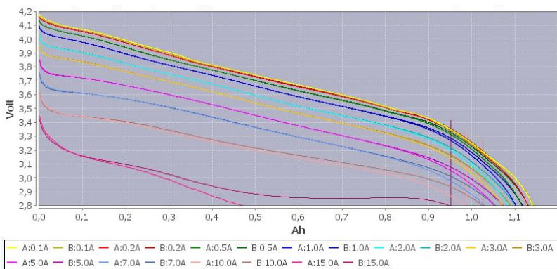
Charakterystyka rozładowania ogniwa IMR18350 KEEPPOWER
