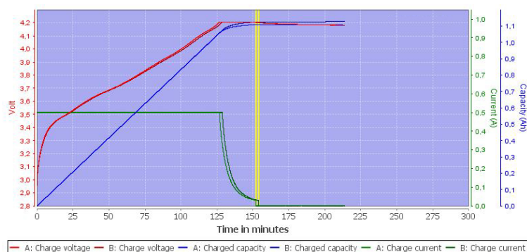
Charakterystyka ładowania ogniwa IMR18350 KEEPPOWER
